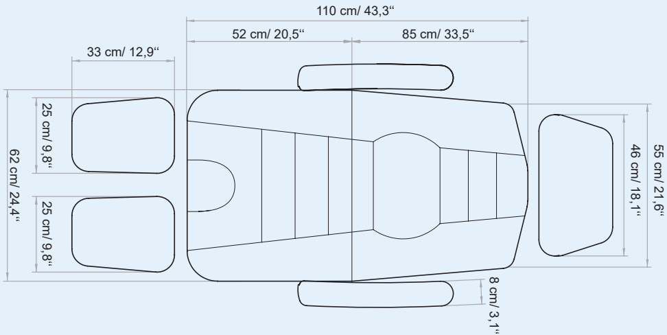
PODO 5 PODO MIX 3M
